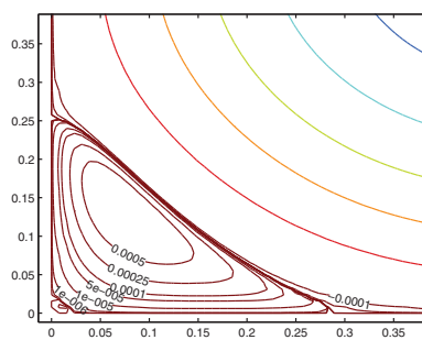
FIG. 5.10. Left eddy , Re = 5000 .
