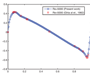
FIG. 5.12. v(x, 0.5) , Re = 5000 .
