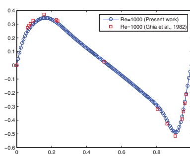
FIG. 5.6. v(x, 0.5) , Re = 1000 .
