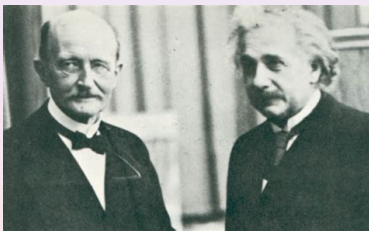
Planck and Einstein
